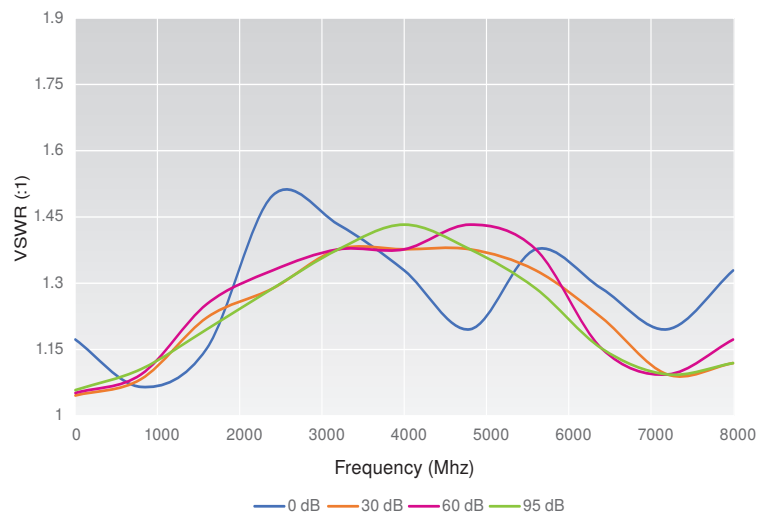
Output VSWR
